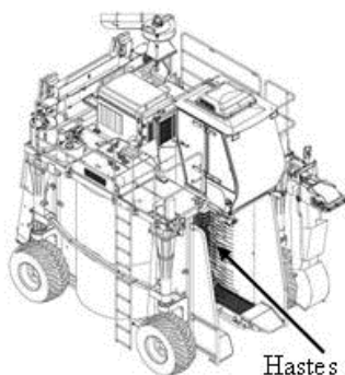
Hastes vibratórias
